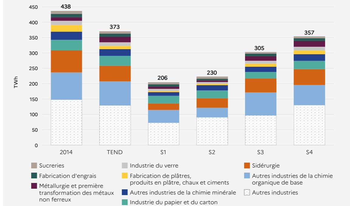
Graphique 16 Répartition des consommations d'énergie (dont matières premières) en 2014 et en 2050, par scénario et par type d'industrie (IGCE et autres)
